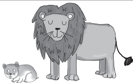
hamster
